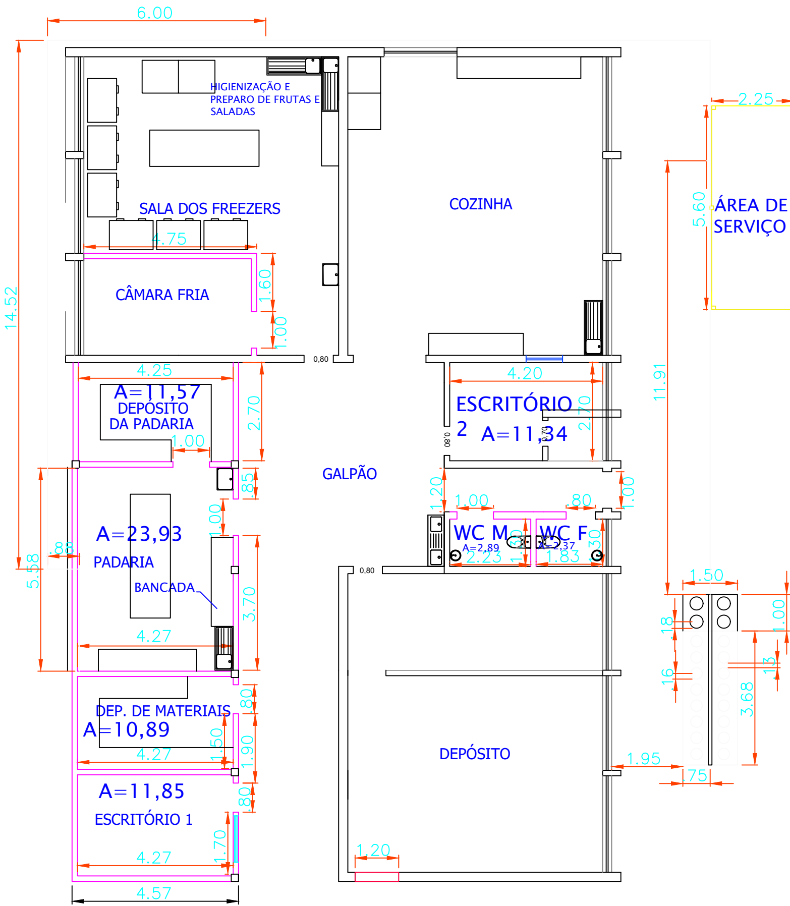
PLANTA BAIXA COZINHA PILOTO ESCALA: 1:100
