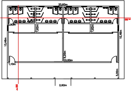
PLANTA BAIXA
