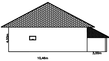
FACHADA LATERAL
