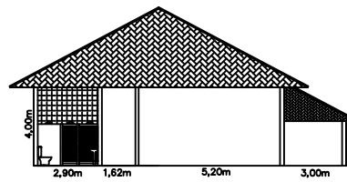
CORTE BB
