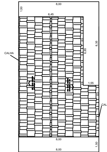
COBERTURA ESCALA 1:100
