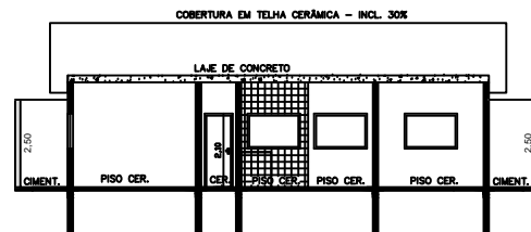
CORTE A-A ESCALA 1:100
