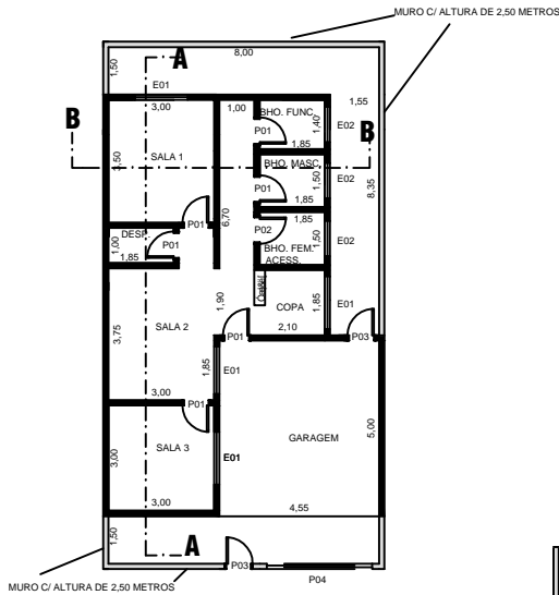
PLANTA BAIXA ESCALA 1:100
