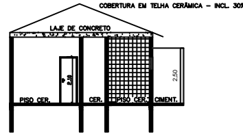
CORTE B-B ESCALA 1:100
